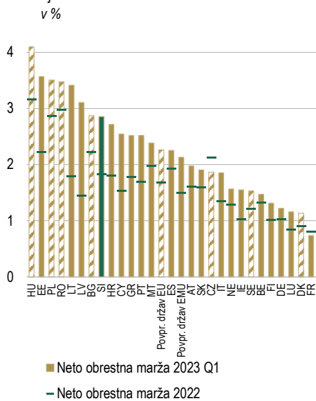
Slika 2.25: Neto obrestna marža in rast neto obrestnih prihodkov po državah EU
