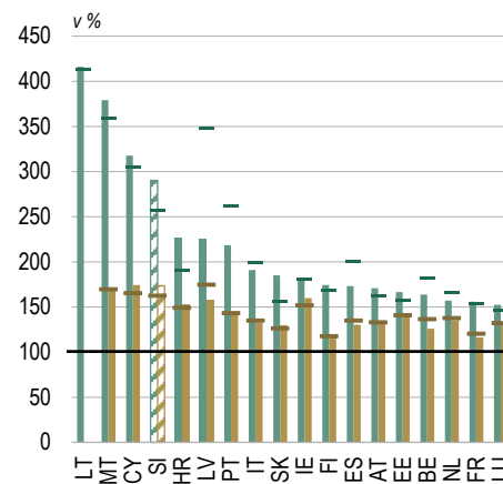
Količnik likvidnostnega kritija in količnik neto stabilnega financiranja po državah evrskega območja
