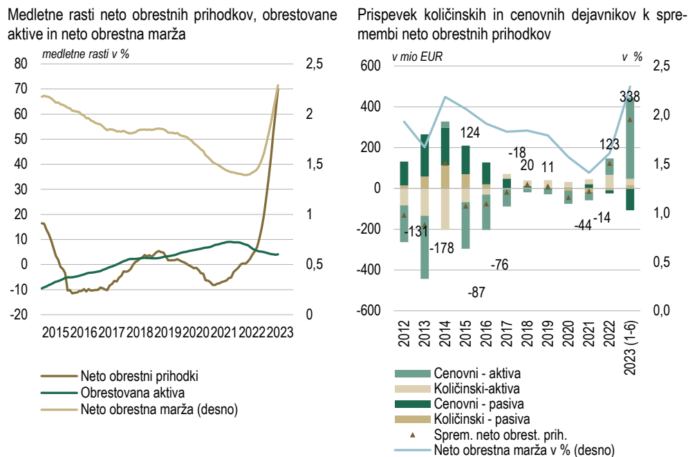
Slika 2.22: Neto obrestna marža in prispevek količinskih ter cenovnih učinkov k spremembi neto obrestnih prihodkov
