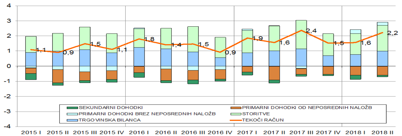
STRUKTURA TEKOČEGA RAČUNA v % BDP (BDP je vsota štirih četrtletj BDP do obravnavanega četrtletja)
