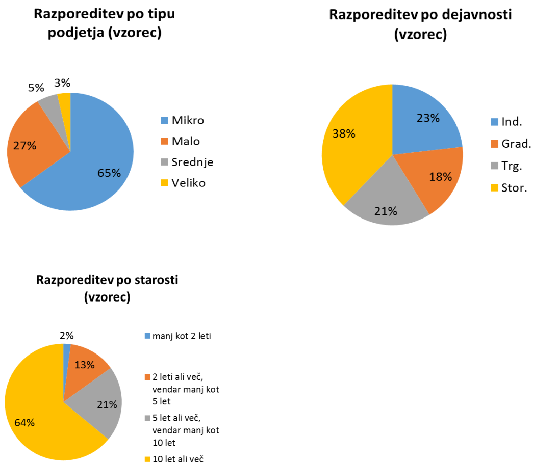
Slika 1: Deskriptivna statistika vzorca
