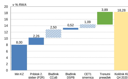
Slika 2.10: Sestava kapitalске zahteve, konsolidirana osnova
