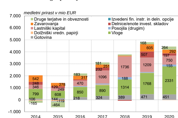
Slika 3.6: Struktura prirasta finančnega premoženja gospodinjstev
