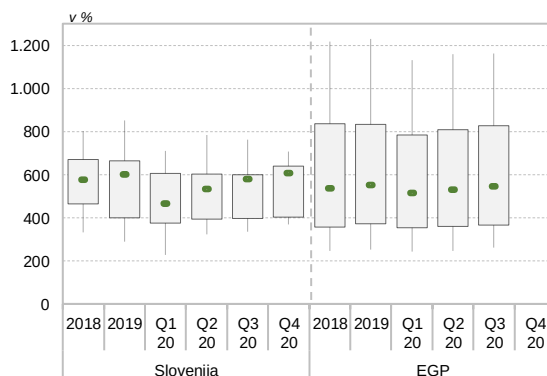
Slika 4.12: Kapitalska ustreznost glede na minimalni konsolidirani zahtevani kapital (zav.)
