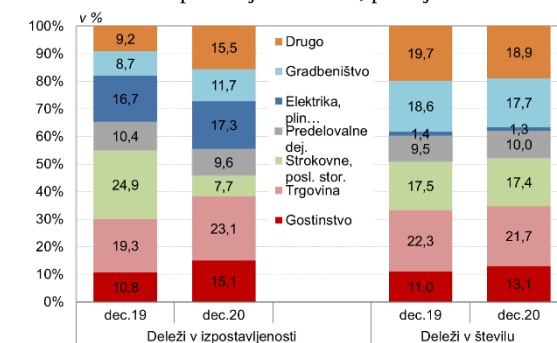
Slika 3.18: Struktura blokiranih transakcijskih računov nefinančnih družb glede na število in izpostavljenost bank, po dejavnostih
