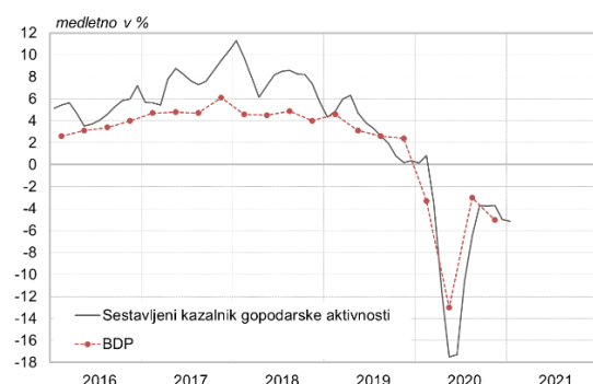
Slika 1.7: Sestavljeni kazalnik gospodarske aktivnosti in realni BDP
