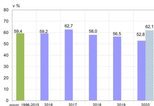
Slika 1.51: Kazalnik razmerja med operativnimi stroški in bruto dohodkom (Cost-to-income ratio); v letu 2020 tudi brez učinka združitve dveh bank
