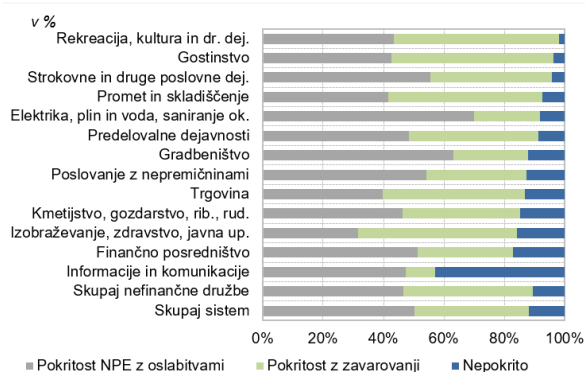
Slika 1.39: Struktura pokritosti NPE z oslabitvami in zavarovanji po dejavnostih konec leta 2020
