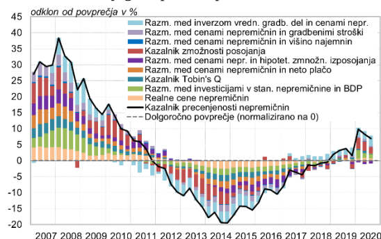
Slika 1.73: Kazalnik precejnosti nepremičnin in njegove podkomponente
