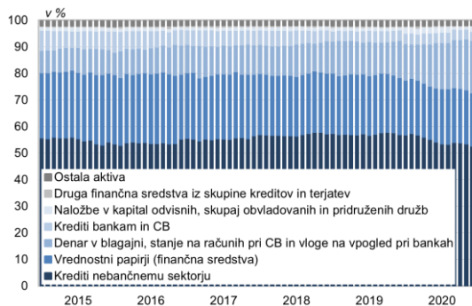
Slika 1.104: Struktura bilance bančnega sistema – aktiva
