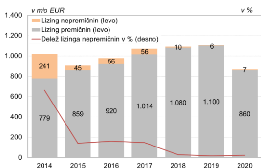
Slika 4.1: Novoodobreni lizinški 115 posli
