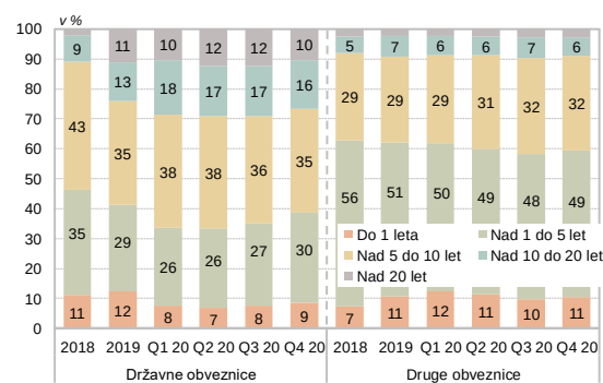
Slika 4.10: Struktura naložb (po)zavarovalnic v obveznice po ročnosti
