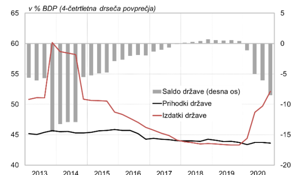
Slika 1.12: Prihodki, izdatki in saldo države
