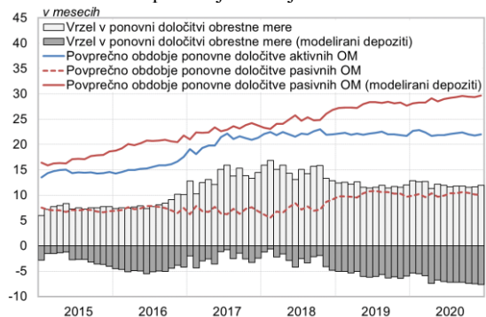
Slika 1.102: Primerjava vrzeli v ponovni določitvi obrestne mere med aktivnimi in pasivnimi obrestno občutljivimi pozicijami upoštevajoč zunajbilanco
