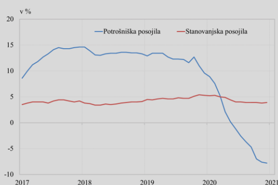
Slika 5.6: Medletne kreditne rasti za potrošniška in stanovanjska posojila
