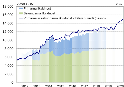
Slika 2.17: Gibanje primarne in sekundarne likvidnosti
